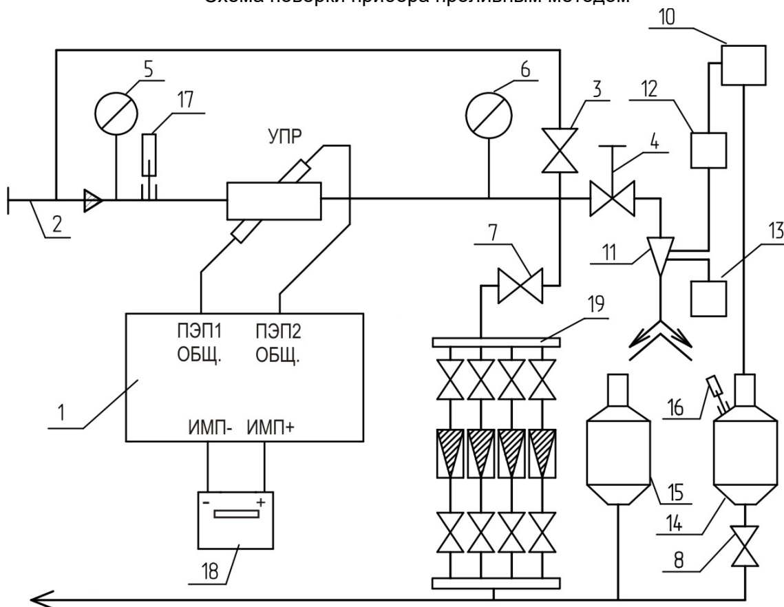
Схема поверки прибора проливным методом
